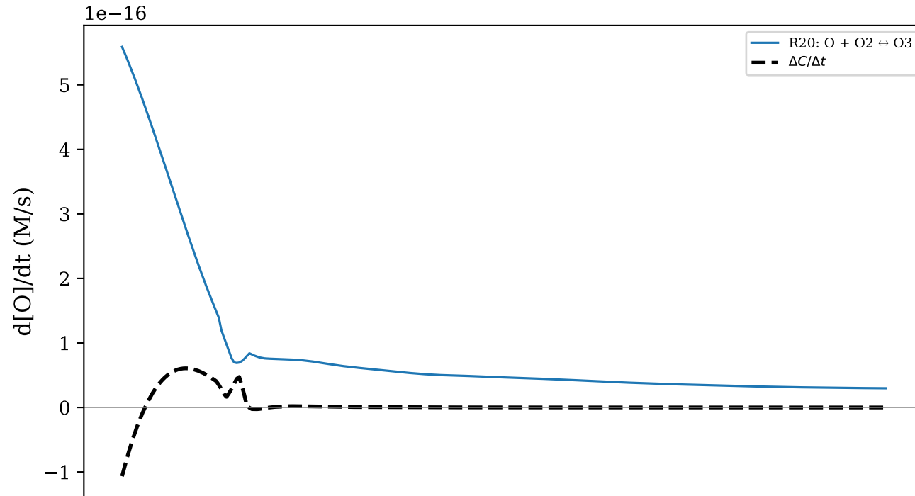
(a) O [final=-0.01 pM]
